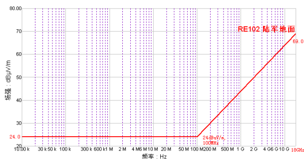
图 6 陆军地面 RE102 场强极限值曲线
