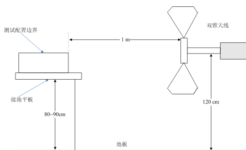
图 3 双锥天线定位图
