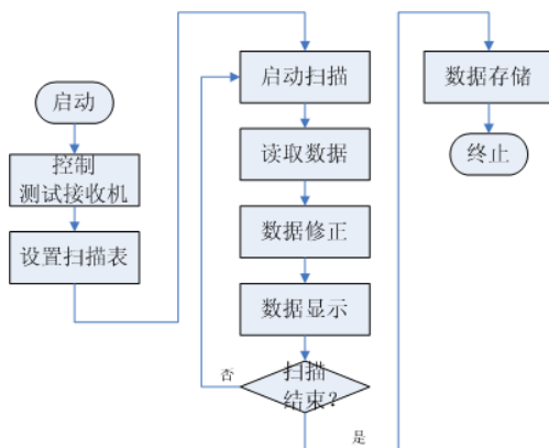
图 5 传导发射测试流程
