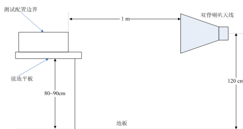
图 4 双脊喇叭天线定位图
