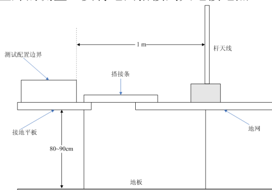
图 2 拉杆天线定位图
