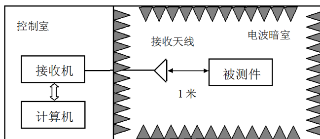
图 1 RE102 测试布置
